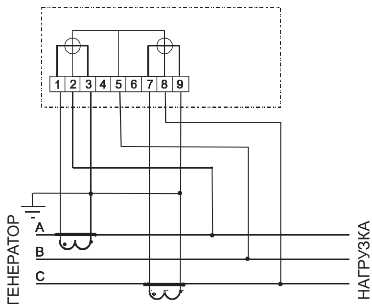
Рисунок Б.6 – Схема включения двухэлементного счетчика в трехпроводную сеть без трансформаторов напряжения
