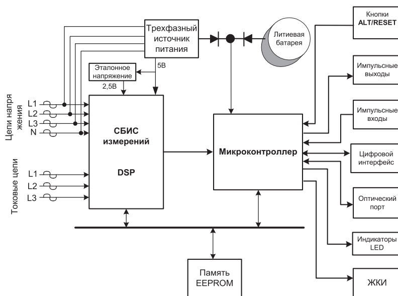
Рисунок 3 – Структурная схема счетчика Альфа А1700
