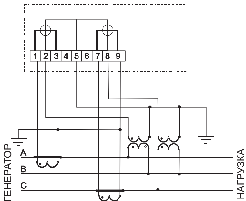
Рисунок Б.4 – Схема включения двухэлементного счетчика в трехпроводную сеть с двумя трансформаторами напряжения
