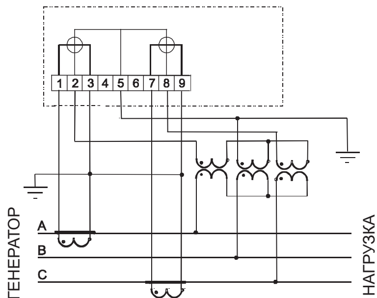
Рисунок Б.5 – Схема включения двухэлементного счетчика в трехпроводную сеть с тремя трансформаторами напряжения и заземленной фазой В
