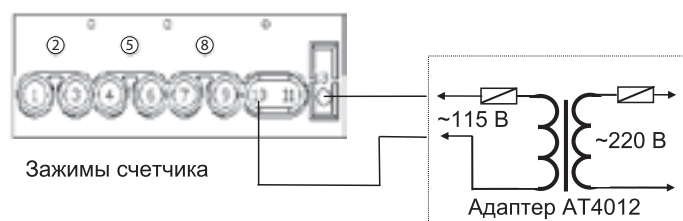
Рисунок Б.7 – Схема подключения адаптера резервного питания АТ4012 к счетчику
