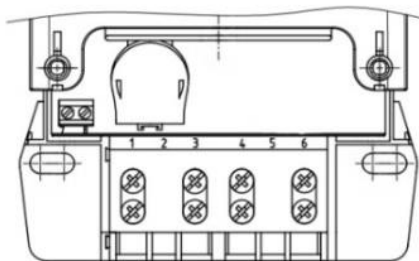
Рисунок 3.2 – Нумерация контактов счетчика СЕ208ВУ S7
