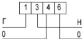
Рисунок 4.1а. Схема подключения счетчика
