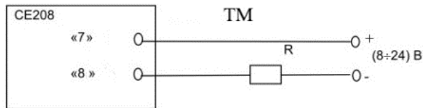
Рисунок 4.2 – Подключение импульсного выхода
