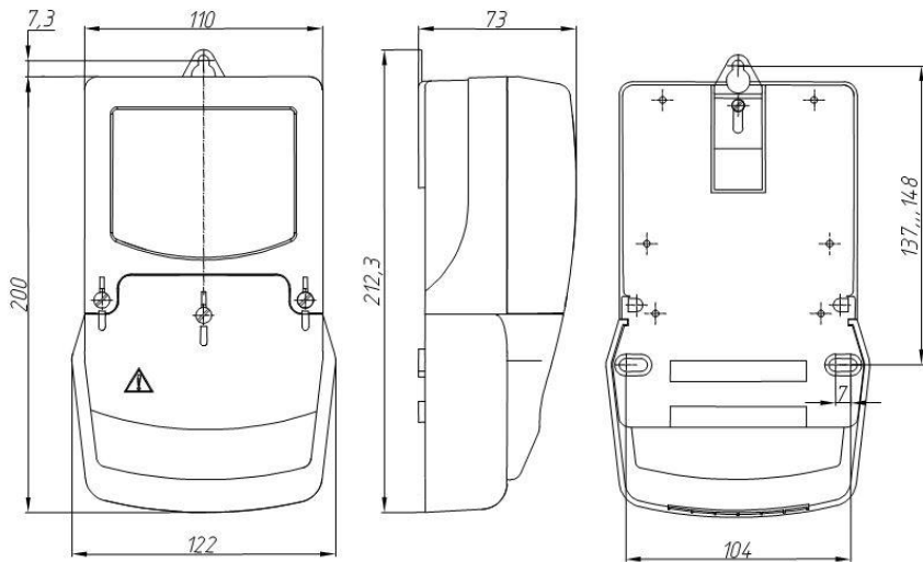
Рисунок А.1 - Счетчик в корпусе S7
