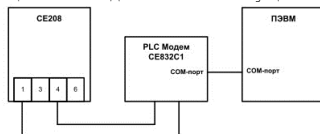
Рисунок 4.4 – Схема подключения счетчика СЕ208 к ПЭВМ через PLC-интерфейс
