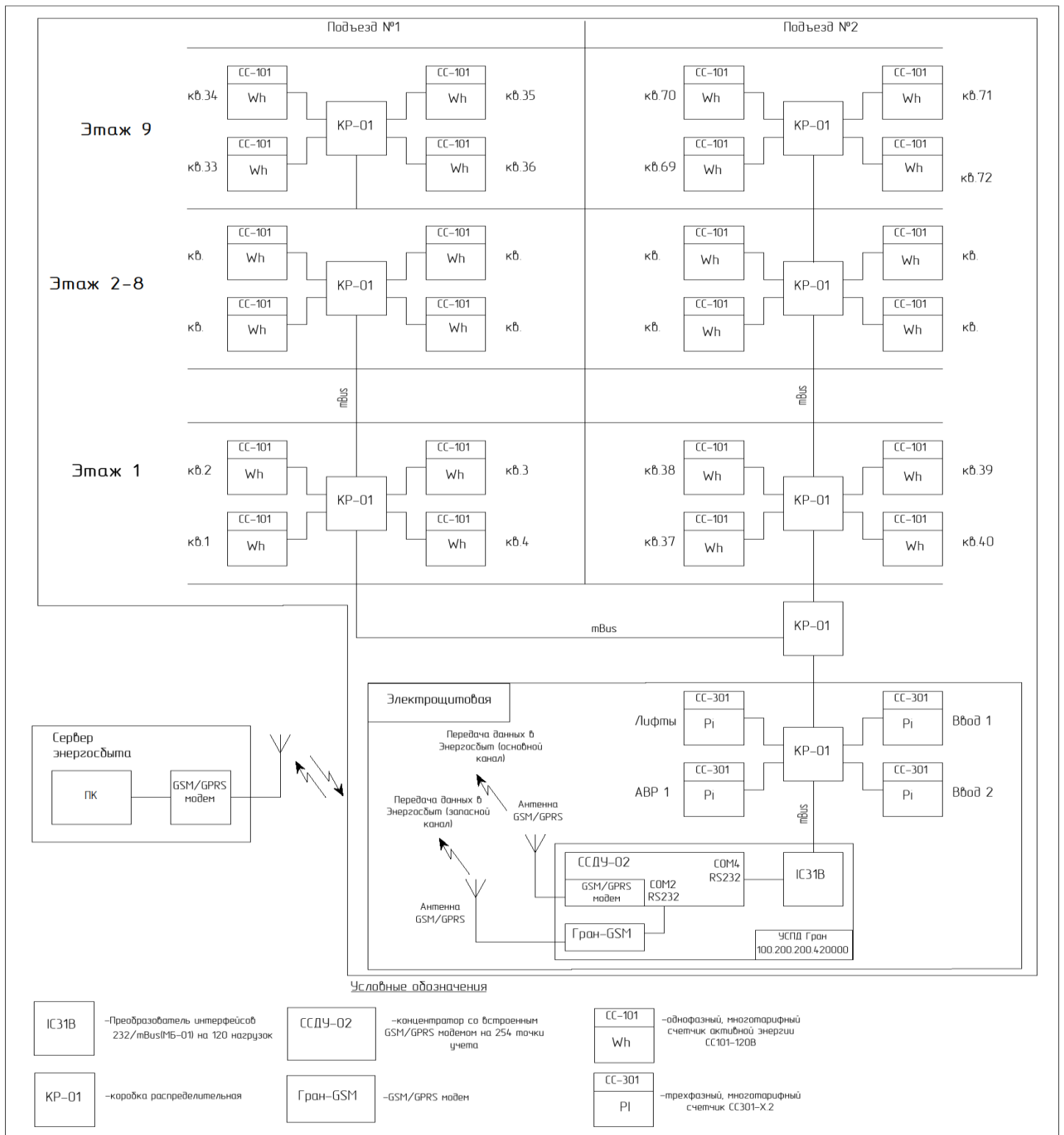
Рисунок Д.1 – Пример построения системы АСКУЭ для 9-ти этажного 72-х квартирного жилого дома с использованием УСПД «Гран» для учета электроэнергии с интерфейсом M-Bus на 72 точки учета
